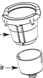
Assemblage du support à K-Cup
